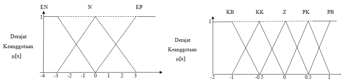
Gambar 3. Fungsi keanggotaan error dan dError suhu
