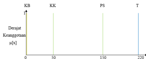
Gambar 4. Fungsi Keanggotaan keluaran suhu (VAC)
