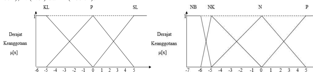
Gambar 5. Fungsi Keanggotaan error dan deror kelembaban.
