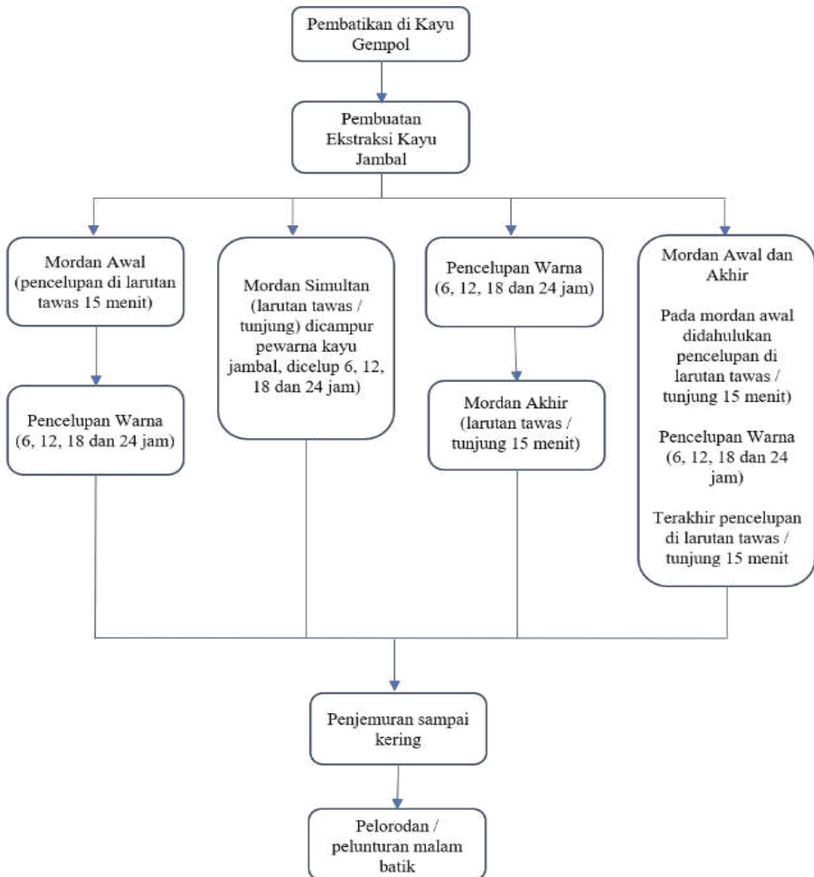
Gambar 3 Bagan Eksperimen
