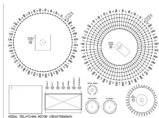
Gambar 10. Kertas Pola (template) pengukur kepersisian sudut
