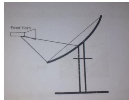
Gambar 4. Bentuk Offset Feed
