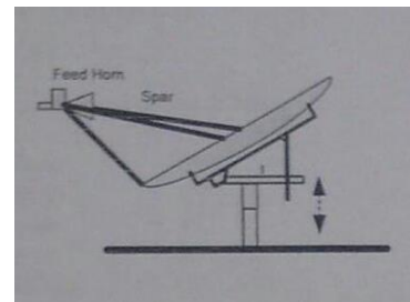
Gambar 8. Bentuk pemasangan spar pada antenna
