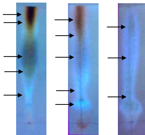
Gambar 4 Pola kromatogram satu arah menggunakan eluen BAW. Tanda panah menunjukkan senyawa yang berbeda untuk tiap organ.
