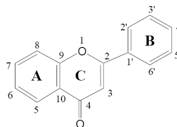
Gambar 2. Struktur umum flavonoid [20]
