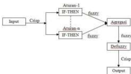
Gambar 2.1 Diagram blok FIS
