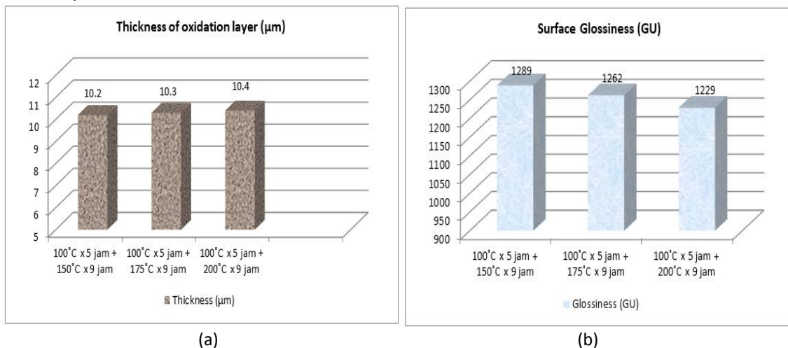
Gambar 5. Hasil Pengukuran Thickness of Oxidation Layer (a) dan Hasil Pengukuran Surface Glossiness dari ketiga percobaan.
