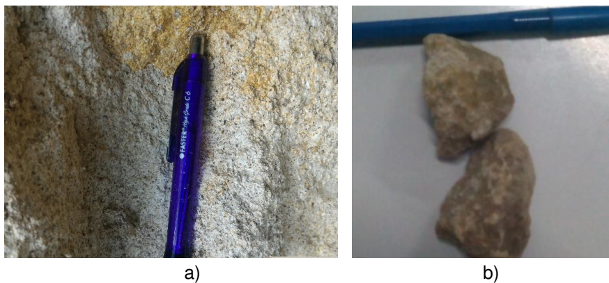
Gambar 3. Litologi Daerah Penelitian terdiri dari: a). Batugamping dan b). Batupasir kuarsa.
