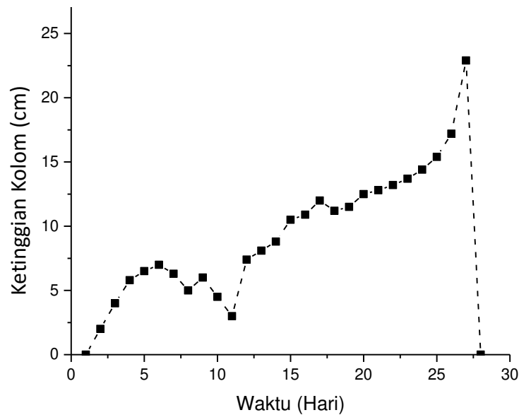
Gambar 4. Hubungan antara masa retensi dengan ketinggian kolom air.
