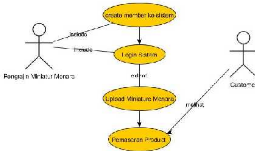
Gambar 3. Usecase Diagram Social Media Marketing untuk pengrajin miniature menara kodus.
