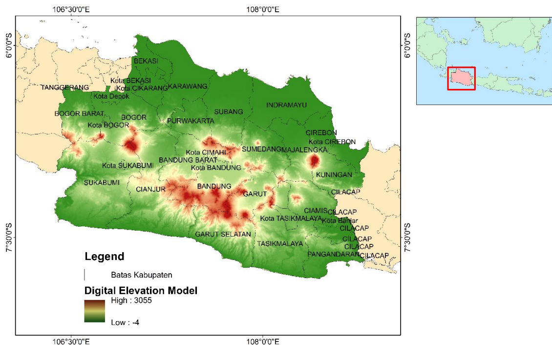
Gambar 1 Bentuk topografi permukaan Provinsi Jawa Barat berdasarkan digital elevation model (DEM) yang diunduh dari https://earthexplorer.usgs.gov/ .
