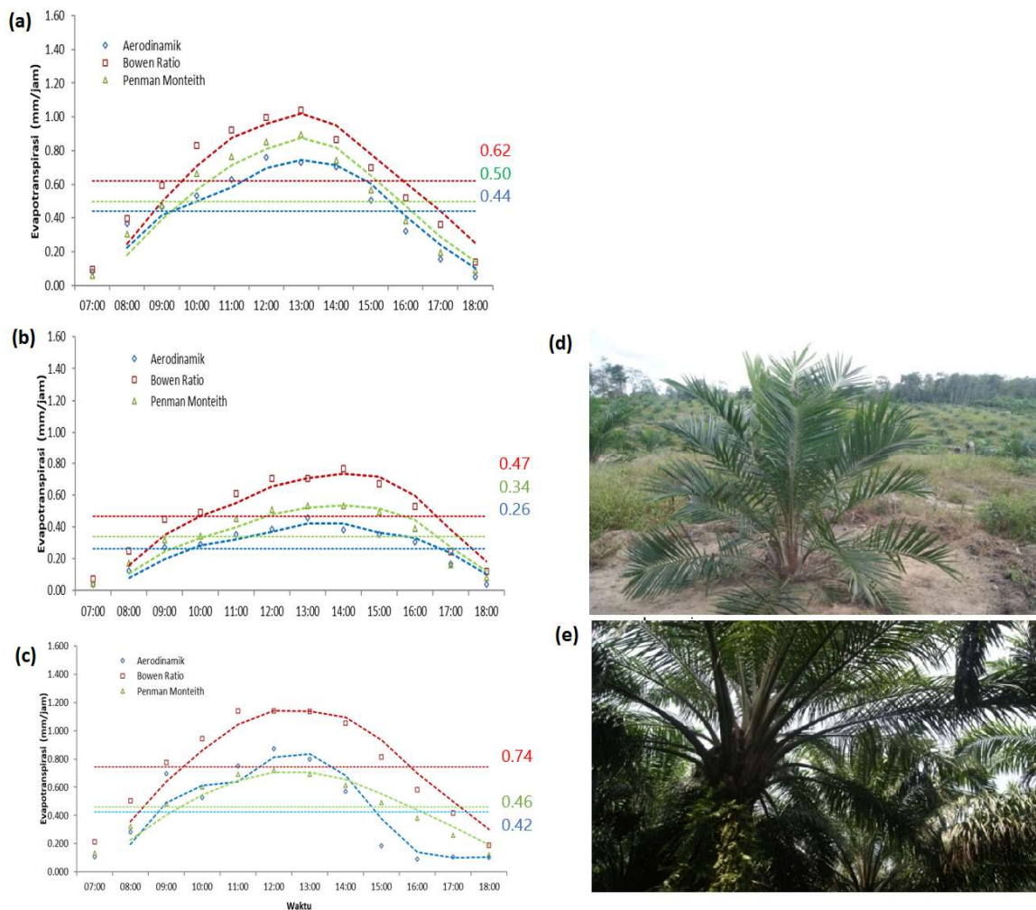
Gambar 3 Evapotranspirasi pertanaman kelapa sawit: (a) umur dua tahun Desa Pempa Air, Jambi (tanpa mempertimbangkan persyaratan fetch ), (b) sawit umur dua tahun Desa Pempa Air, Jambi (dengan mempertimbangkan persyaratan fetch ), (c) sawit umur sepuluh tahun di PT Perkebunan Nusantara VIII, Kebun Cimulang, Jawa Barat (dengan mempertimbangkan persyaratan fetch ). Tanaman kelapa sawit pada umur dua tahun di Desa Pempa Air (d), dan sawit umur sepuluh tahun di PT Perkebunan Nusantara VIII (e)
