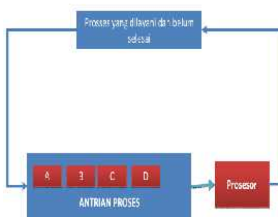
Gambar 3. Penjadwalan Proses
