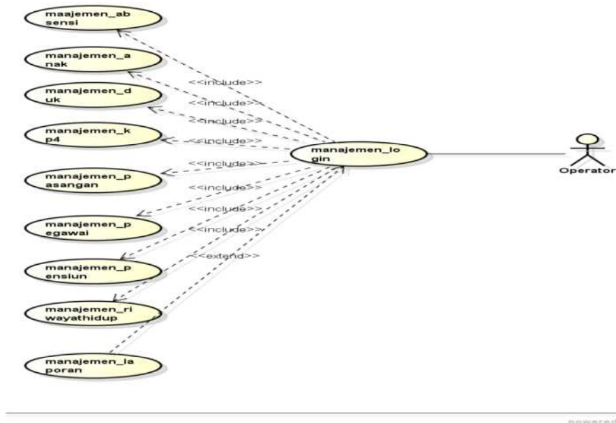
Gambar 1 Use-Case Diagram Sistem Informasi Kepegawaian
