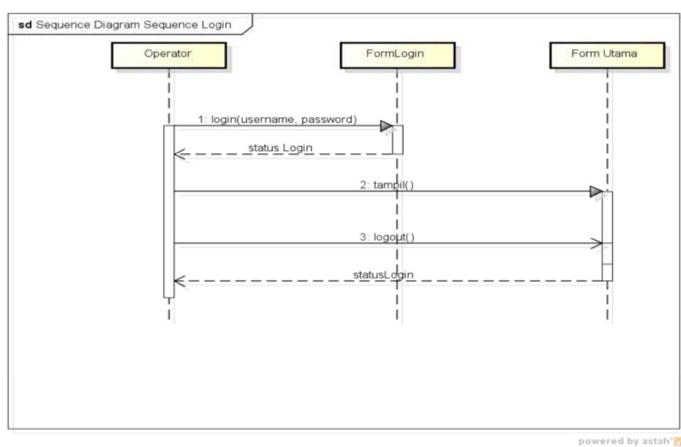
Gambar 3 Sequence Diagram Login Sistem Informasi Kepegawaian
