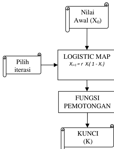
Gambar 2. Proses urutan pembangkit kunci
