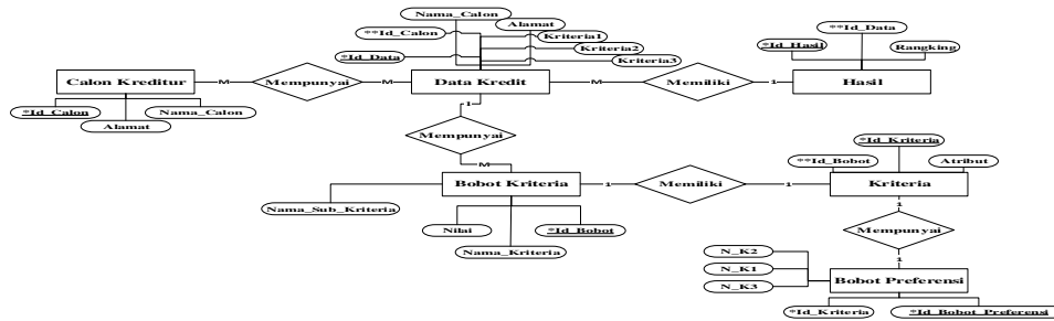
Gambar 4. ERD
