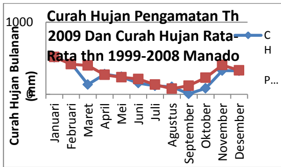
Gambar 6. Curah Hujan Pengamatan thn 2009 dan Curah Hujan Rata-Rata Tahun 1999- 2008 Manado
