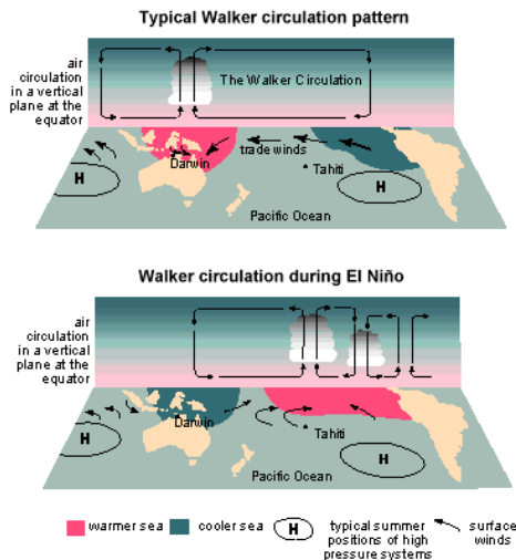
Gambar 1. Pola Sirkulasi Walker Keadaan Normal Dan Keadaan El-Nino
