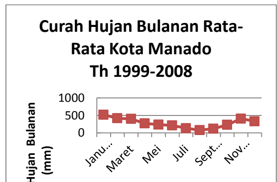
Gambar 3. Curah Hujan Bulanan Rata-rata Manado Thn 1999-2008
