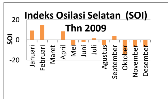
Gambar 5. Indeks Osilasi Selatan Thn 2009
