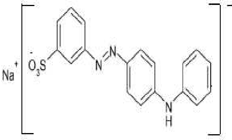
Gambar 1 : Struktur kimia metanil yellow
