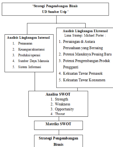
Gambar 2.2 Kerangka Berpikir
