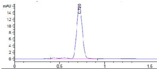
Gambar 4. Kromatogram klorpirifos pada laju alir fasa gerak 0,70 mL/menit
