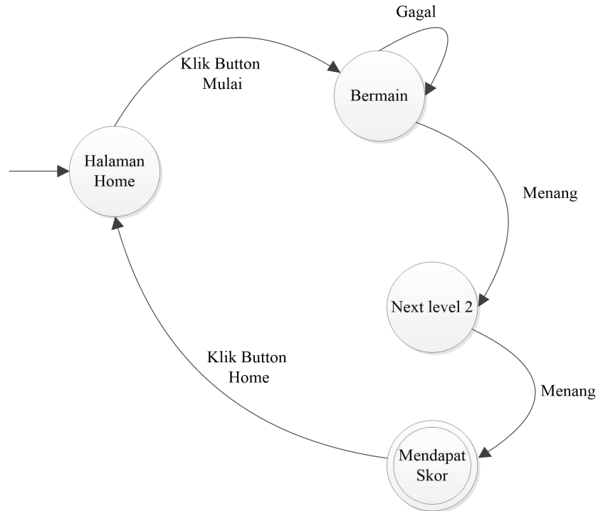
Gambar 1. FSM Pada Game Perakitan Komputer
