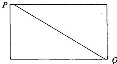
Gambar 3 Jarak terpendek dari P ke Q
