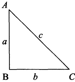
Gambar 1 Segitiga siku-siku ABC
