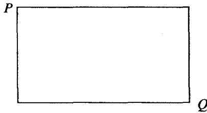
Gambar 2 Suatu taman berbentuk persegi panjang
