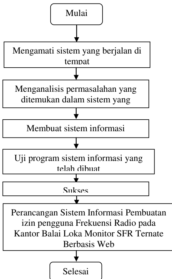
Gambar 1. Kerangka Berpikir
