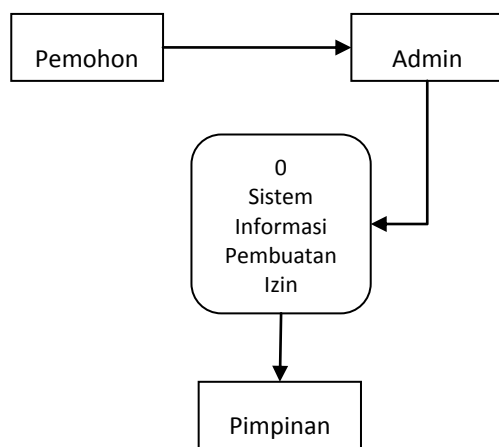
Gambar 4. Diagram Konteks
