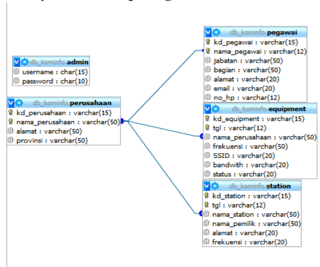
Gambar 8. ERD
