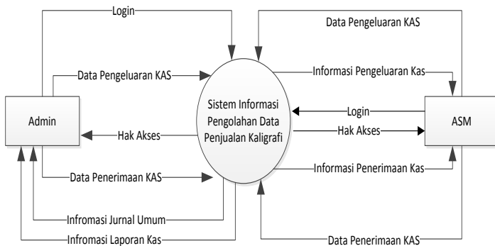
Gambar 5. Diagram Konteks
