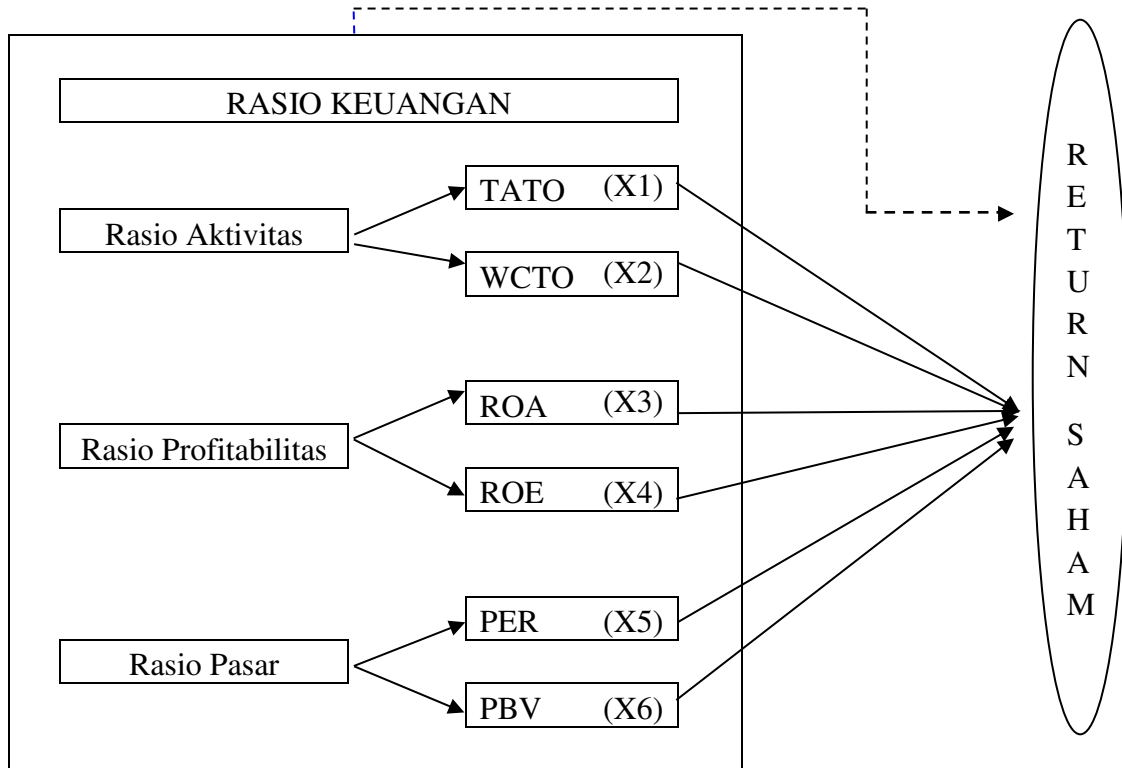
Gambar 1 Kerangka Berpikir
