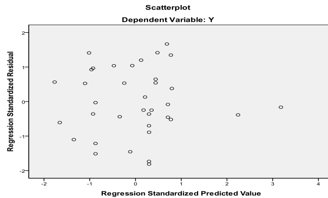
Gambar 2. Uji Heteroskedastisitas
