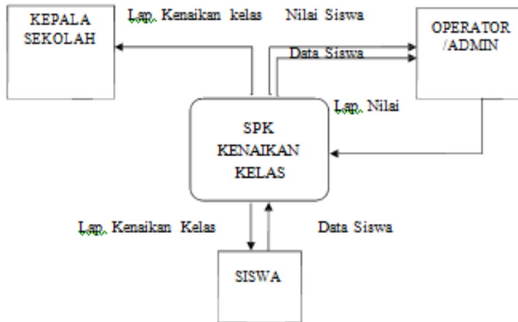
Gambar 3. Diagram Konteks
