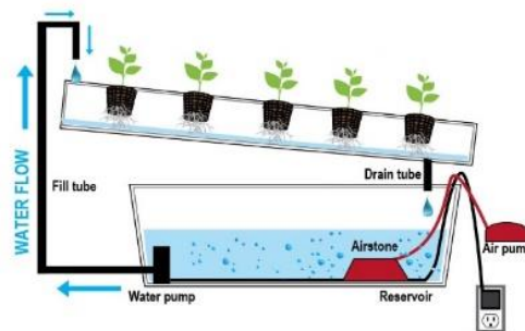
Gambar 1. Sistem Hidroponik NFT ( Nutrient Film Tehnique )
