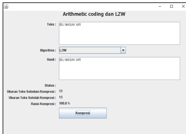
Gambar 3. Tampilan Form Kompresi teks Lempel Ziv Welch (LZW) dan Arithmetic Coding
