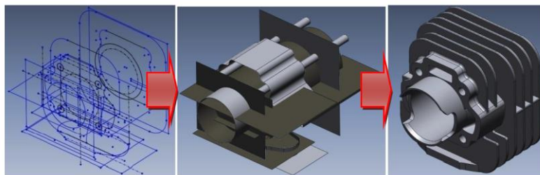
Gambar 8. Pembuatan surface & solid model
