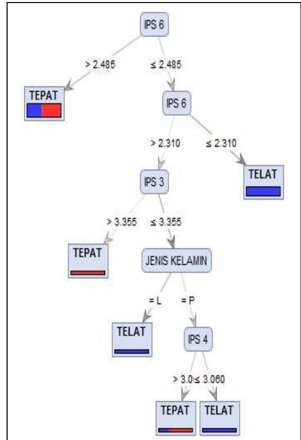
Gambar 2. Pohon keputusan berdasar information gain
