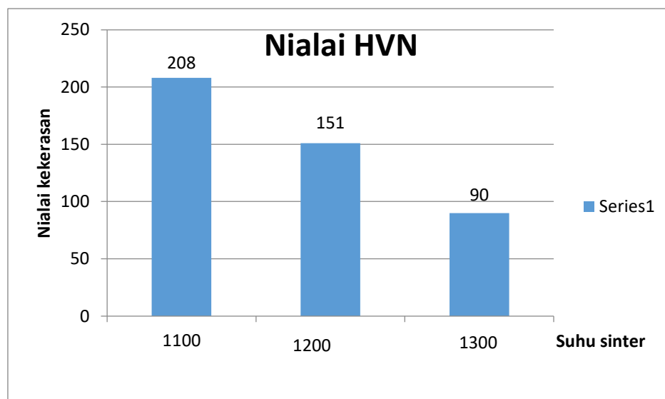
Gambar 7. Grafik Nilai kekerasan hasil sintir
