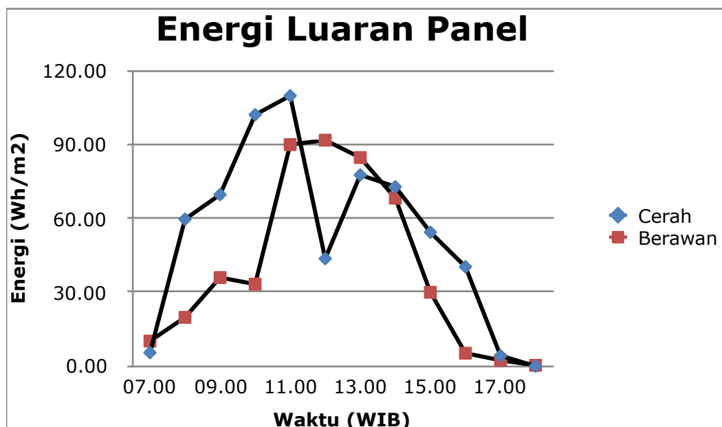
Gambar 2. Keluaran daya panel surya ketika cuaca cerah dan mendung
