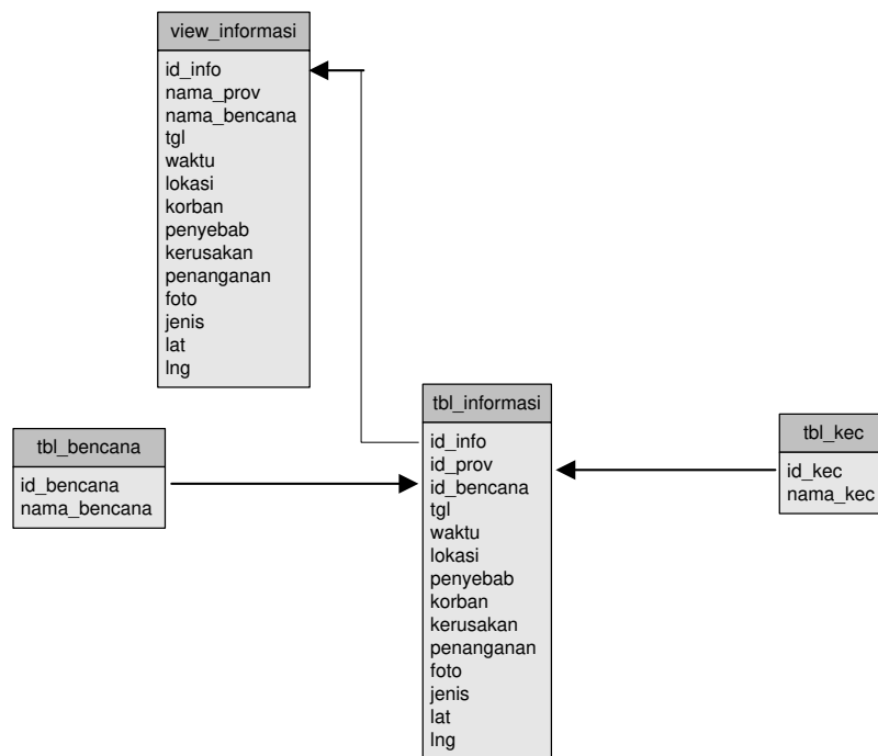
Gambar 4. Relasi Tabel
