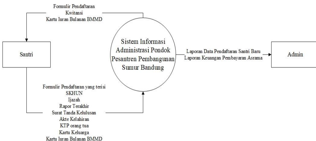
Gambar 1. Diagram Konteks
