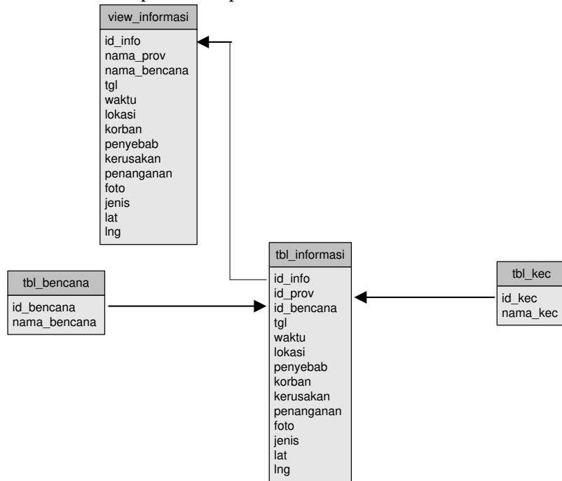
Gambar 4. Relasi Tabel
