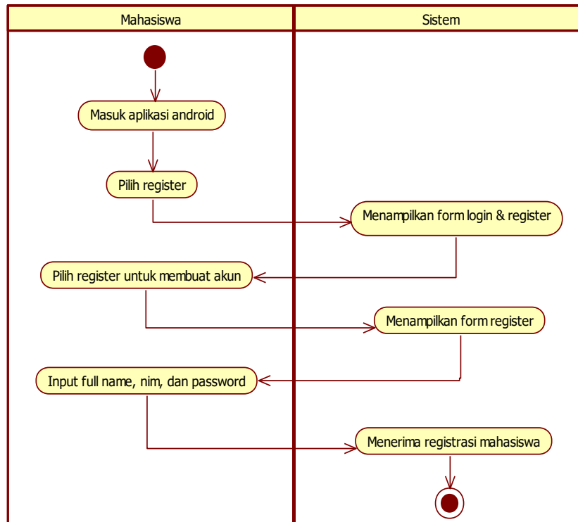
Gambar 4.1 Diagram Aktivitas Register Client yang diusulkan
