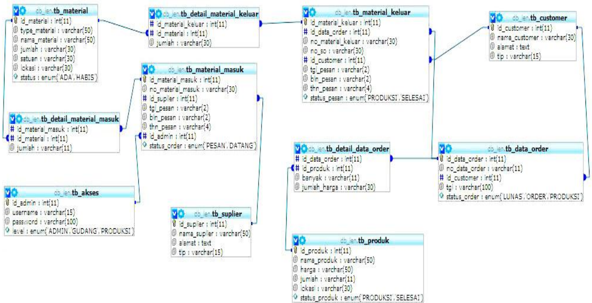
Gambar 8 Gambar Relasi Tabel
