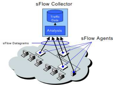
Gambar 2. Teknologi sFlow [6]
