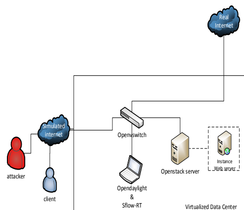
Gambar 4. Topologi Jaringan
