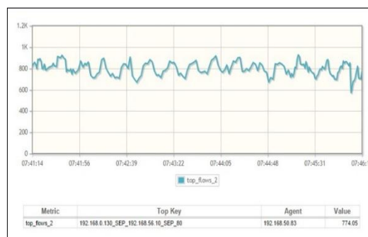
Gambar 9. Grafik sFlow-RT
