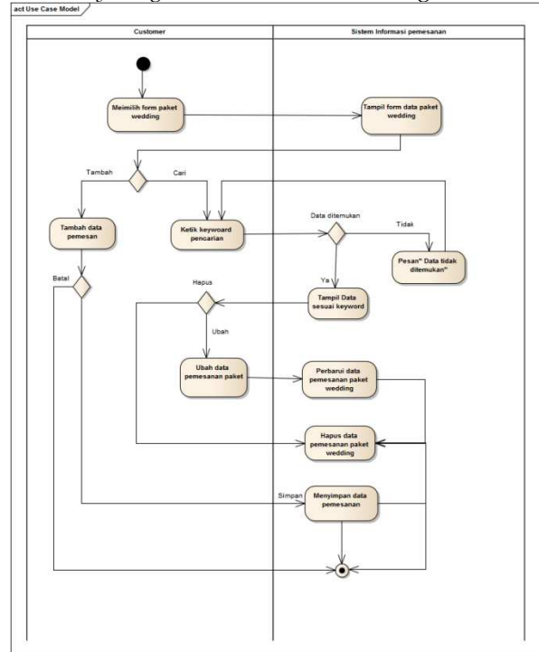
Gambar 3. Activity Diagram Pemesanan
