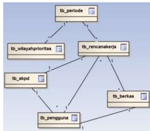
Gambar 1. ERD Sistem Informasi Penanggulangan Kemiskinan
