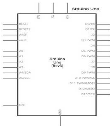
Gambar 10. Skema Arduino
