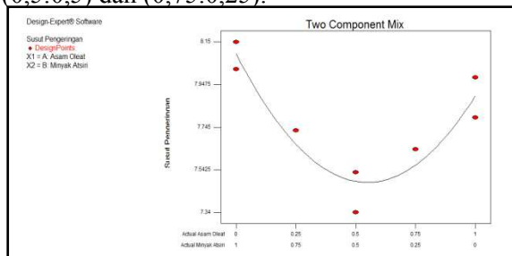
Gambar 4.3 Grafik Hubungan antara Komposisi Campuran Asam Oleat dan Minyak Atsiri Bunga Cempaka Putih terhadap Persentase Susut Pengerangan Matriks Patch
