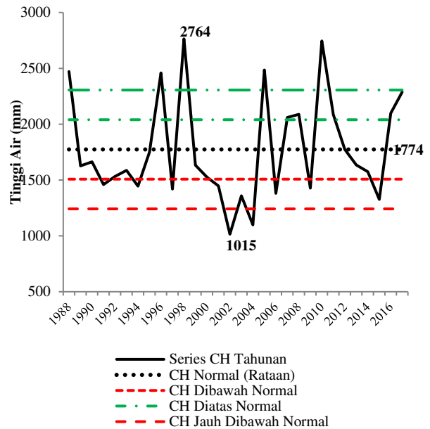
Gambar 1. Distribusi curah hujan (CH) tahunan di Daerah Waeapo
