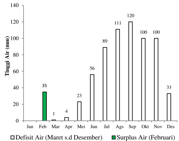
Gambar 3. Periode defisit dan surplus air di Daerah Waeapo pada saat El-Nino
