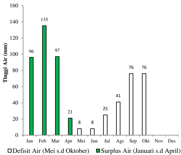
Gambar 2. Periode defisit dan surplus air di Daerah Waeapo pada kondisi curah hujan normal (rata-rata)
