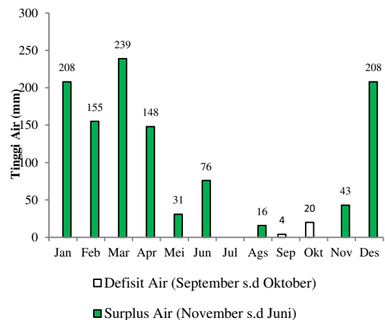
Gambar 4. Periode defisit dan surplus air di Daerah Waeapo pada saat La-Nina
