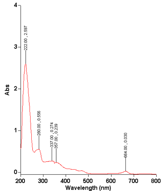
Gambar 1. Spektrum serapan senyawa ekstraksi daun alpukat konsentrasi 100 ppm
