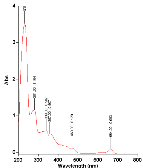
Gambar 2. Spektrum serapan senyawa ekstraksi daun alpukat konsentrasi 200 ppm
