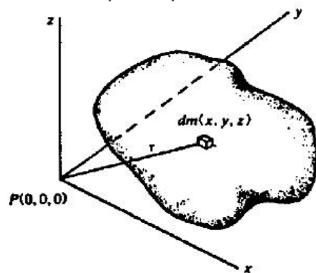
Gambar 2. Potensial massa tiga dimensi [9] Reduksi Data Gravitasi
