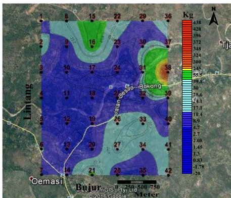
d. Gambar 10. Mikrozonasi indeks kerentanan seismik
