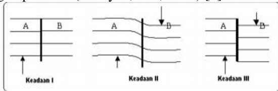
Gambar 1. Skema Deformasi Batuan (Susanto,2011) [3].
