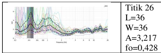
Gambar 4. Salah satu bentuk spektrum HVSr titik 26
