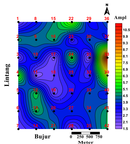
Gambar 6. Kontur amplifikasi
