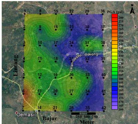
Gambar 9. Mikrozonasi PGA
