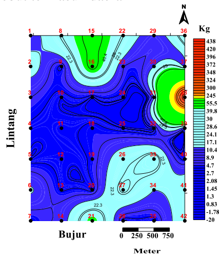
Gambar 7. Kontur Indeks kerentanan seismik
