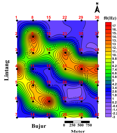
Gambar 5. Kontur frekuensi dominan tanah
