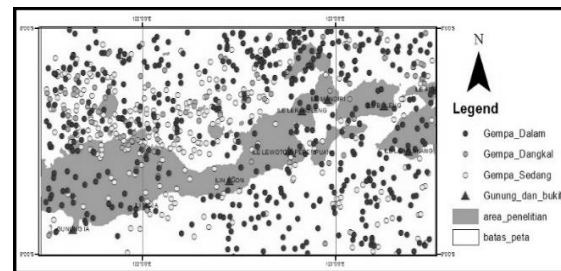
Gambar 6. Peta seismisitas daerah sekitar gunung Lewotobi dan Egon
