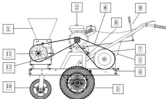
Gambar 1. Skema mesin pengupas kulit kopi berjalan
