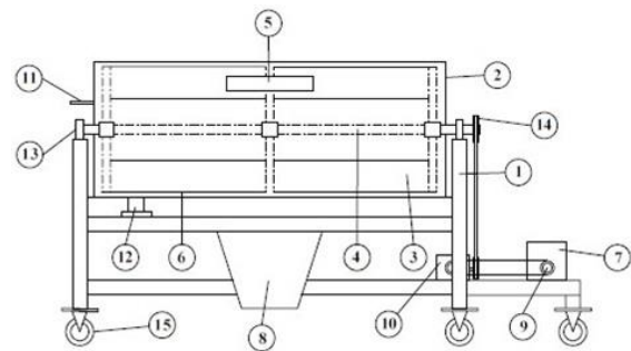
Gambar 2. Skema mesin pencuci biji kopi type batch
