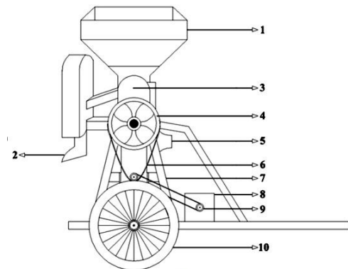
Gambar 3. Skema mesin pengupas biji kopi (huller) berjalan
