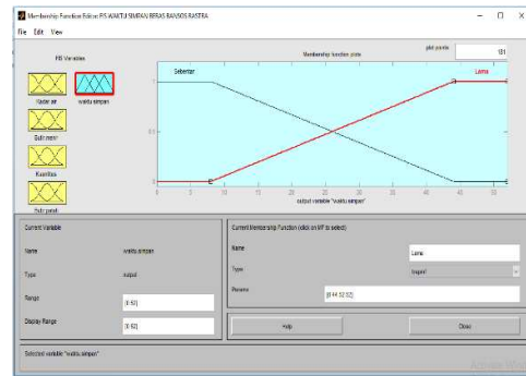
Gambar 16. Himpunan Fuzzy Lama pada Variabel Waktu Simpan
