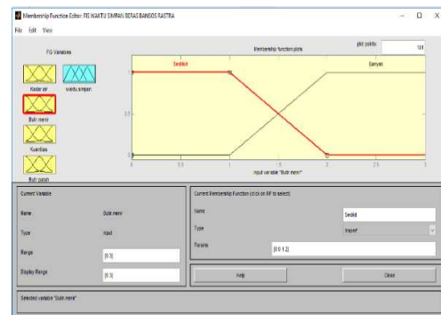
Gambar 9. Himpunan Fuzzy Sedikit pada Variabel Butir Menir
