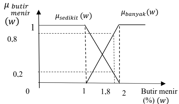
Gambar 2. Grafik Himpunan Fuzzy dan Fungsi Keanggotaan Butir Menir Data 1
