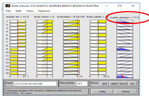
Gambar 19. Hasil Penentuan Waktu Simpan Beras pada Uji Data 2
