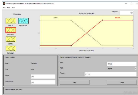
Gambar 10. Himpunan Fuzzy Banyak pada Variabel Butir Menir
