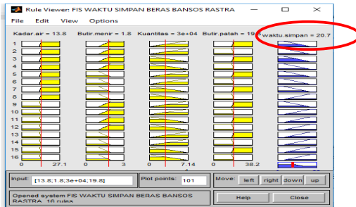
Gambar 18. Hasil Penentuan Waktu Simpan Beras pada Uji Data 1
