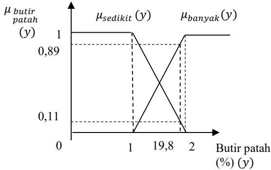
Gambar 4. Grafik Himpunan Fuzzy dan Fungsi Keanggotaan Butir Patah Data 1 (%)( y )
