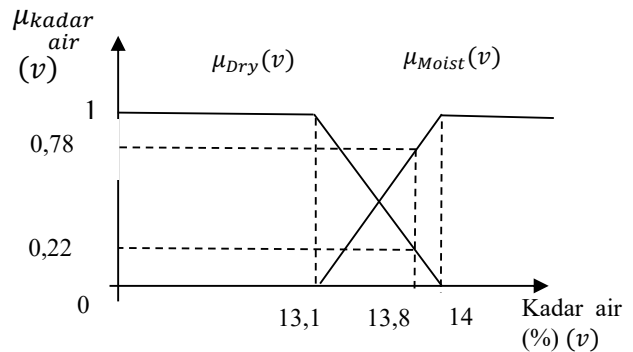
Gambar 1. Grafik Himpunan Fuzzy dan Fungsi Keanggotaan Kadar Air Data 1
