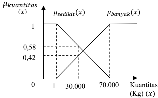
Gambar 3. Grafik Himpunan Fuzzy dan Fungsi Keanggotaan Kuantitas beras Data 1
