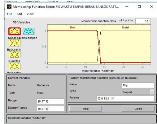
Gambar 7. Himpunan Fuzzy dry pada Variabel Kadar Air
