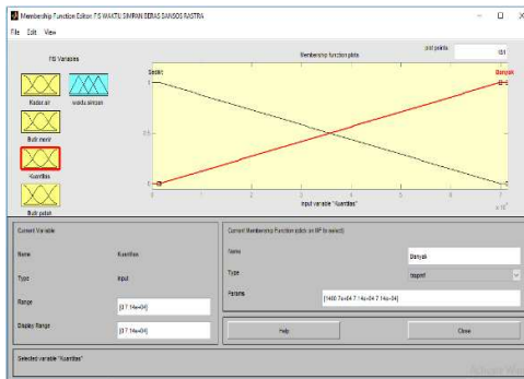
Gambar 12. Himpunan Fuzzy Banyak pada Variabel Kuantitas
